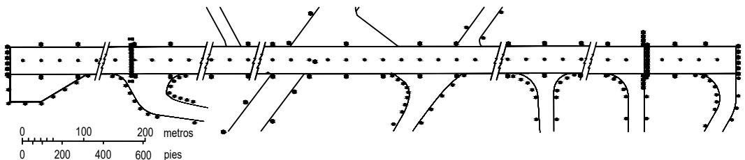
AYUDAS LUMINOSAS RWY 07/25 Y CALLES DE SALIDA
