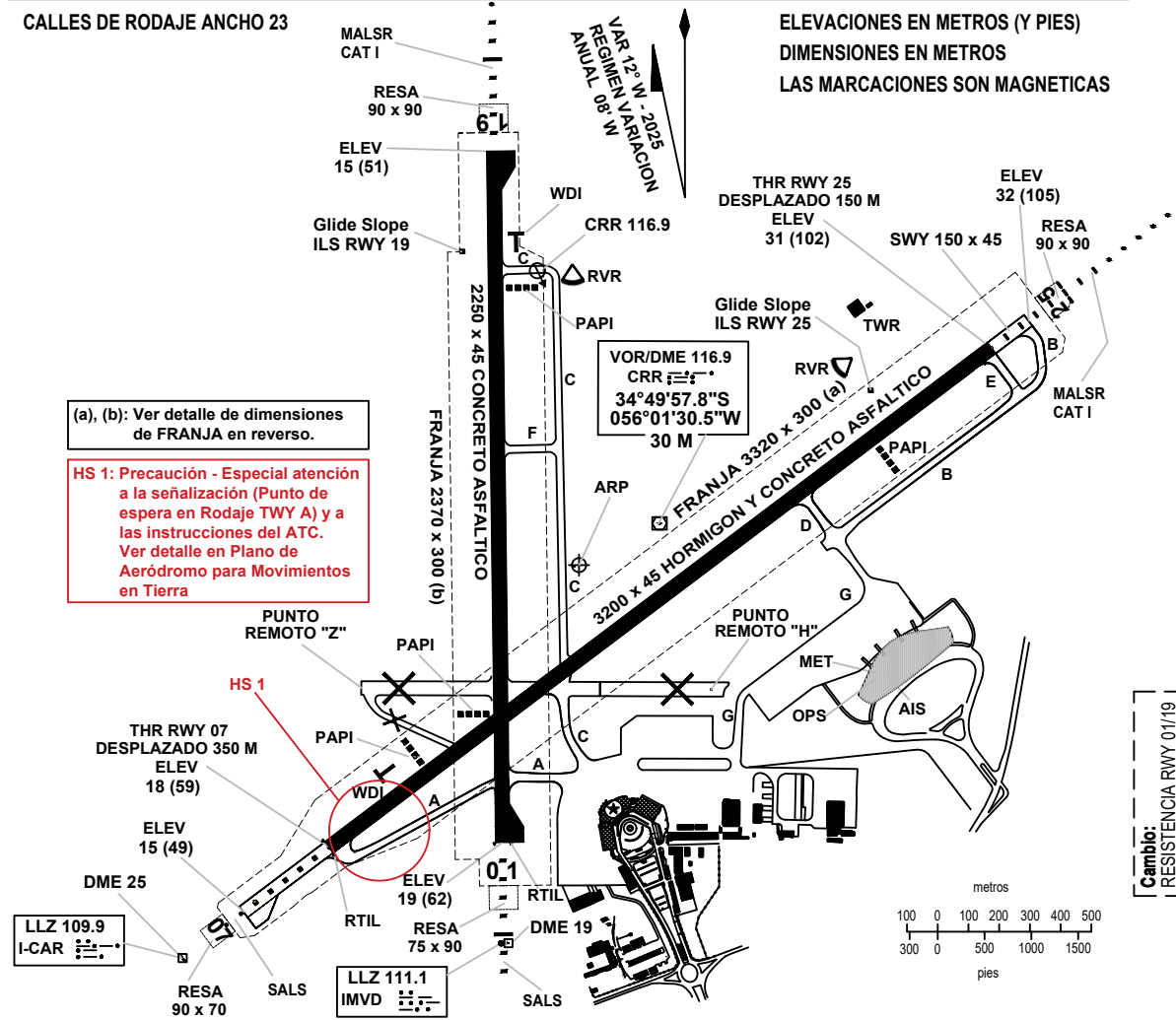
SEÑALES RWY 07/25 Y CALLES DE SALIDA
