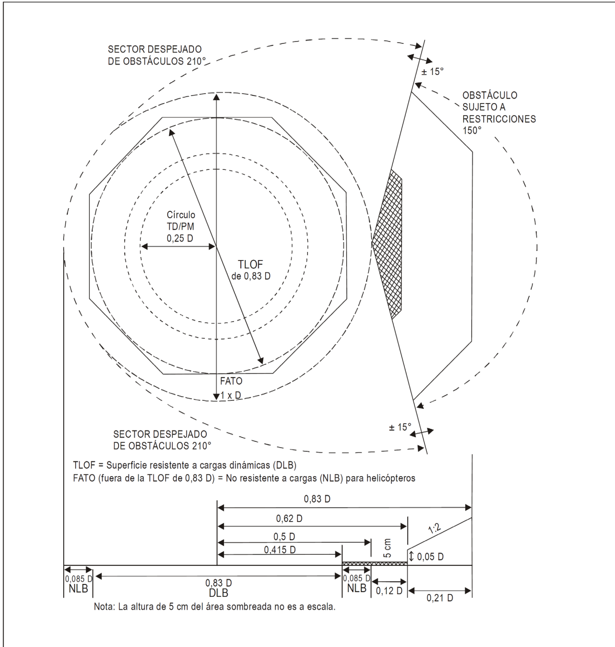
Figura A-4-11 - Sectores y superficies limitadores de obstáculos en heliplateformas para una TLOF de 0,83 D y mayor
