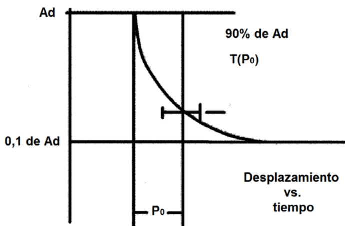
Figura 4.2B Respuesta con amortiguación crítica
